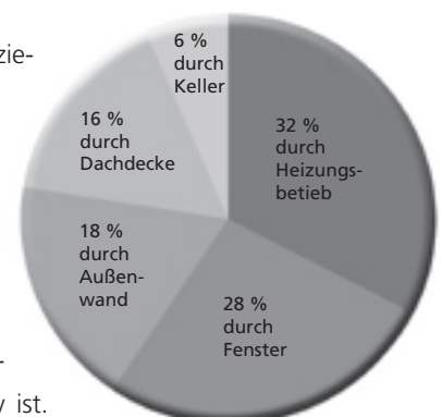
Gesamtwärmeverlust bei einem freistehenden Einfamilienhaus (125 m 2 Wohnfläche)
