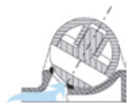
Drehverschluss geschlossen
